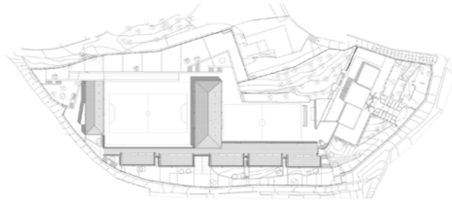
PLANTA BAIXA
