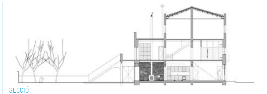
SECCIÓ
